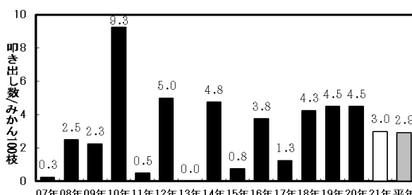
図2 ツヤアオカメムシ越冬数(4カ所平均)
