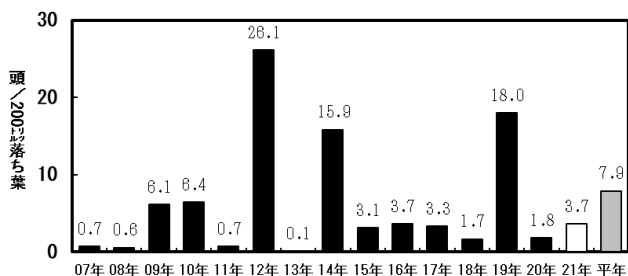
図1 チャバネアオカメムシ越冬数(湯河原・伊勢原)
